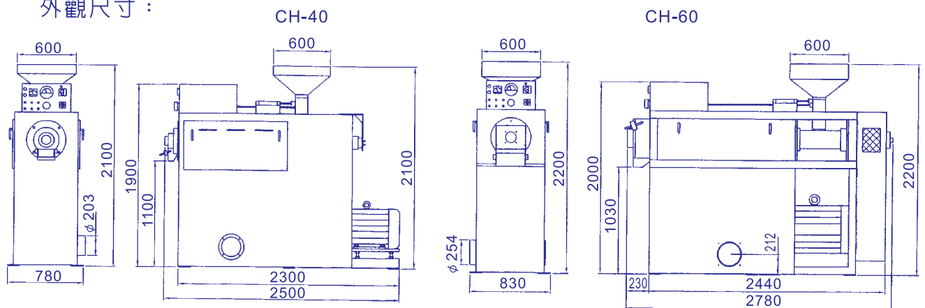
外觀尺寸：
